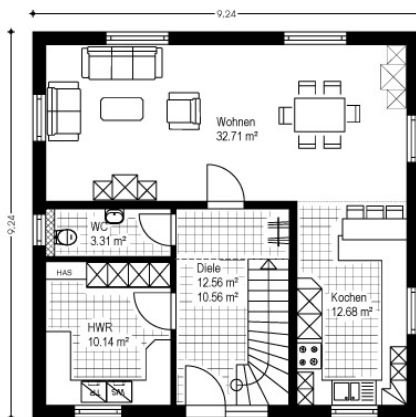
Erdgeschoss
